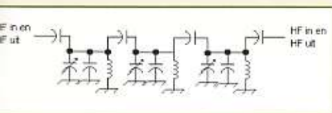
Het HF-filter
